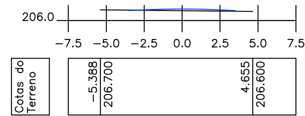
ESTACA S2
