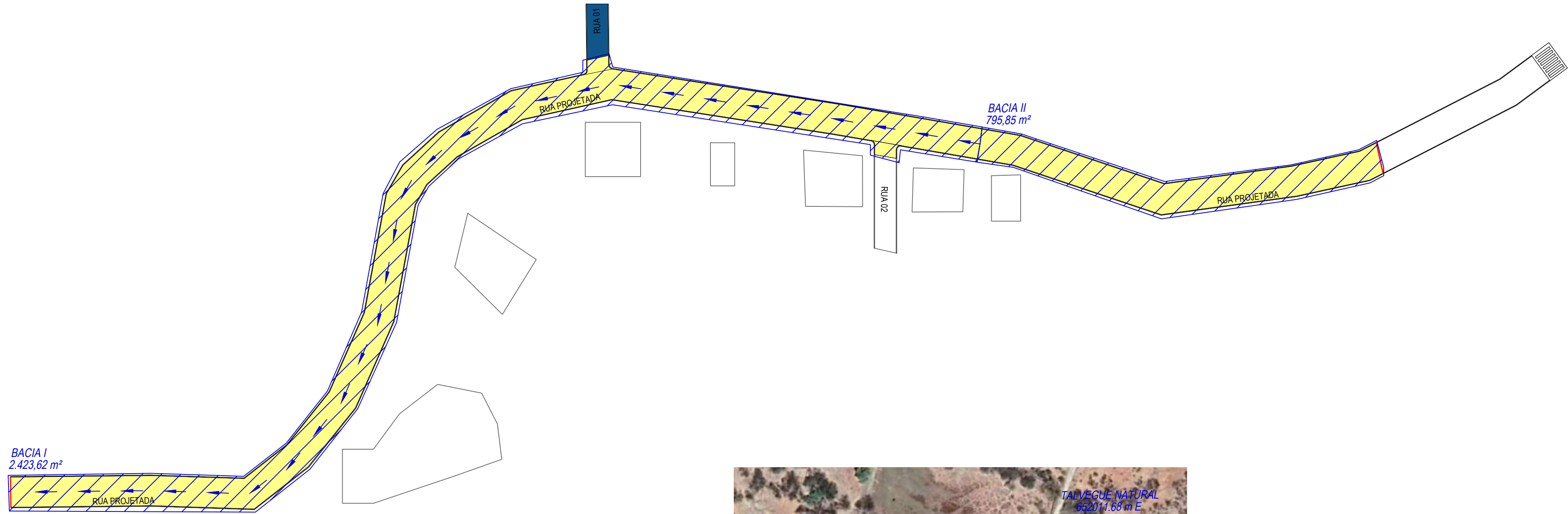
DRENAGEM SUPERFICIAL – R. PROJETADA – SÍTIO MORORÓ escala 1:750
