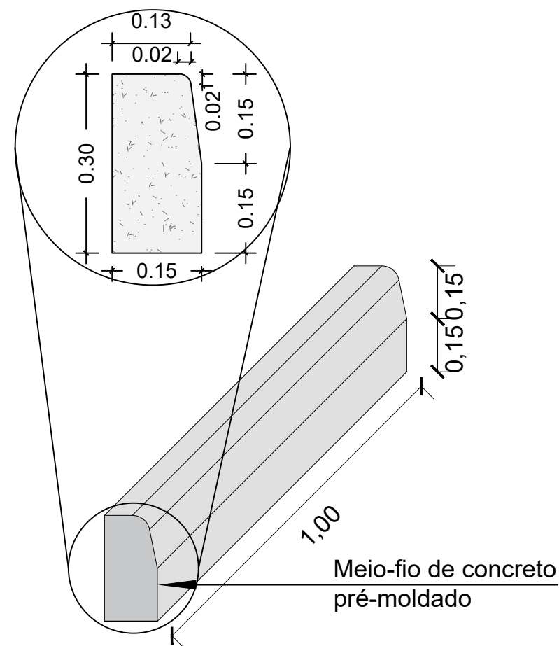
Detalhe 01 - Meio-Fio Pré-Moldado escala 1:15
