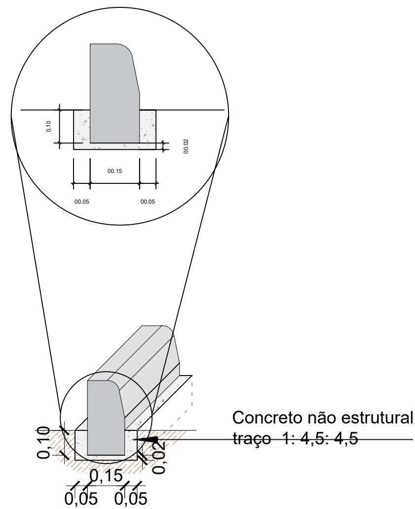
Detalhe 02 - Meio-Fio com Base de Concreto escala 1:15
