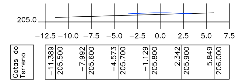
ESTACA S16
