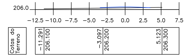
ESTACA S14
