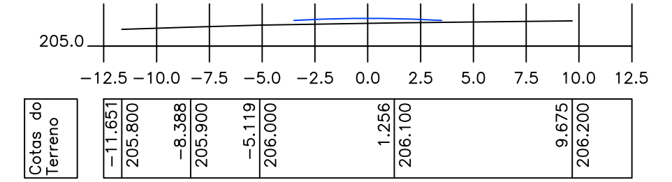
ESTACA S15
