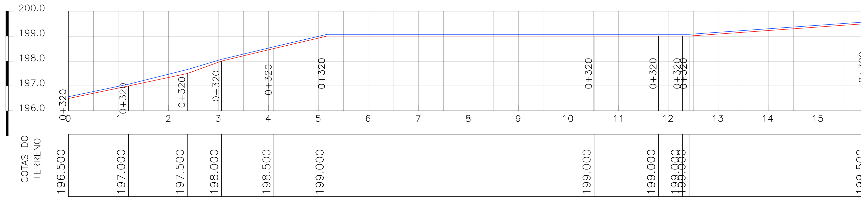
PERFIL LONGITUDINAL DA RUA DA PALHA escala 1/750
