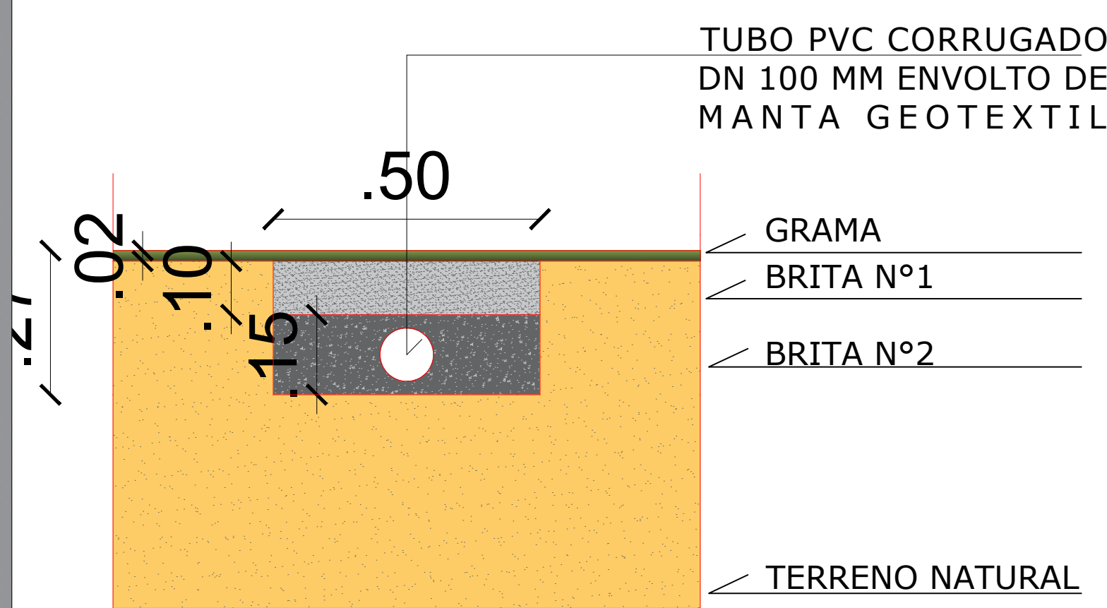
CORTE TRANSVERSAL - DRENAGEM GRAMADO CAMPO ESCALA 1:10
