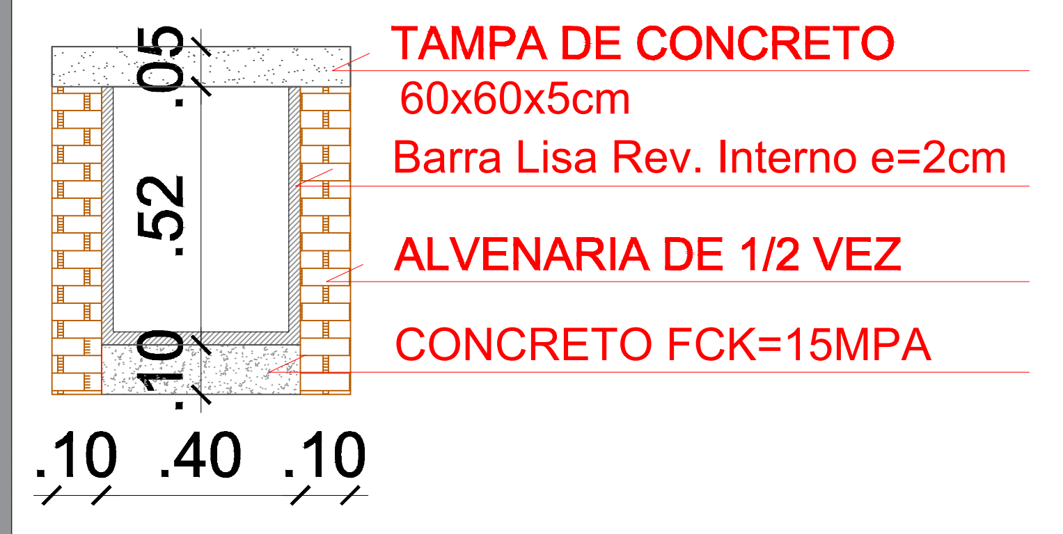
CAIXA DE PASSAGEM SEM ESCALA
