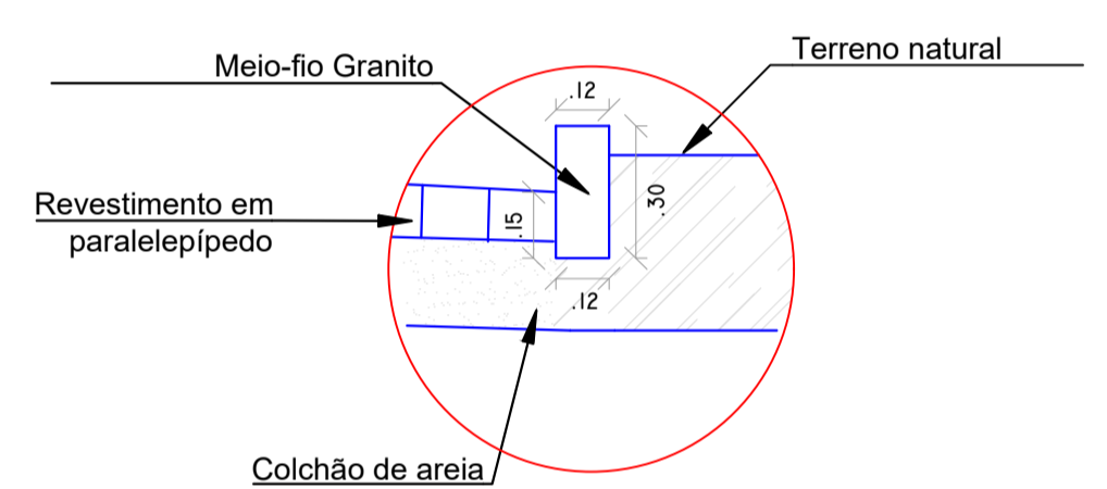
03 DETALHE DO MEIO FIO ESCALA: 1/15
