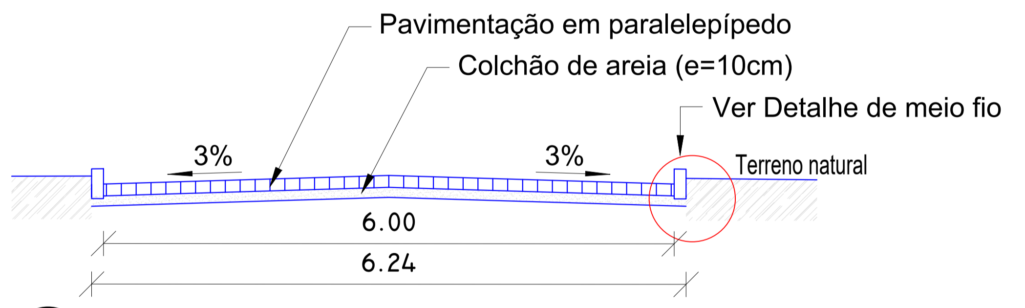
04 SEÇÃO TRANSVERSAL TIPO ESCALA: 1/30
