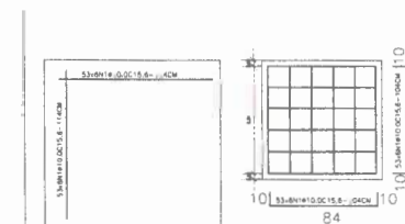
BLOCO DE FUNDAÇÃO - ESTRUTURA FUNCIONAL Escala: 1/25
