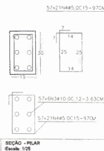
SEÇÃO - PILAR Escala: 1/25
