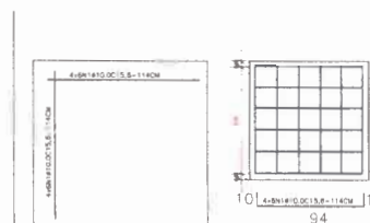
BLOCO DE FUNDAÇÃO - ESTRUTURA CAIXA D'ÁGUA Escala: 1/25
