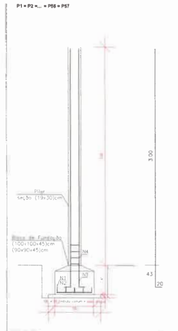
Det. Estrutural: Bloco de Fundação, V. Baldrama e Pilar Escala: 1/25
