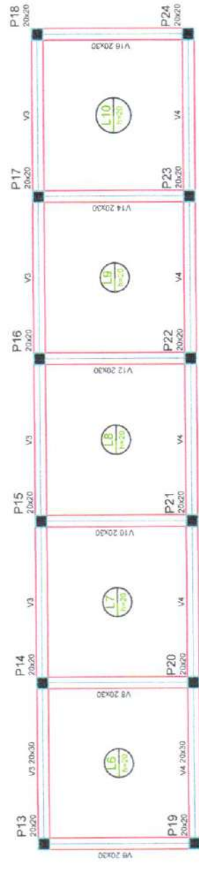
Forma do pavimento pavimento 1 escala 1:50
