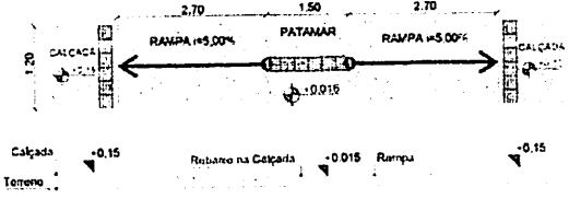
DETALHE DA RAMPA DE ACESSIBILIDADE
