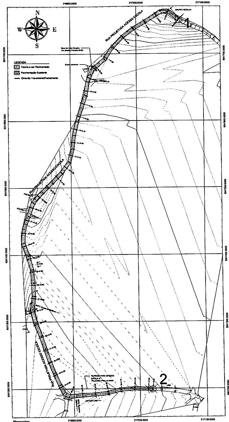
Planimétrico Escala 1:1000
