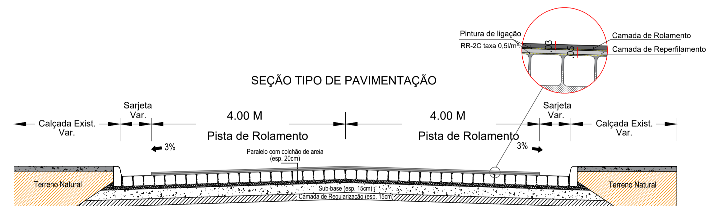
DETALHAMENTO SEÇÃO ESCALA 1/100
