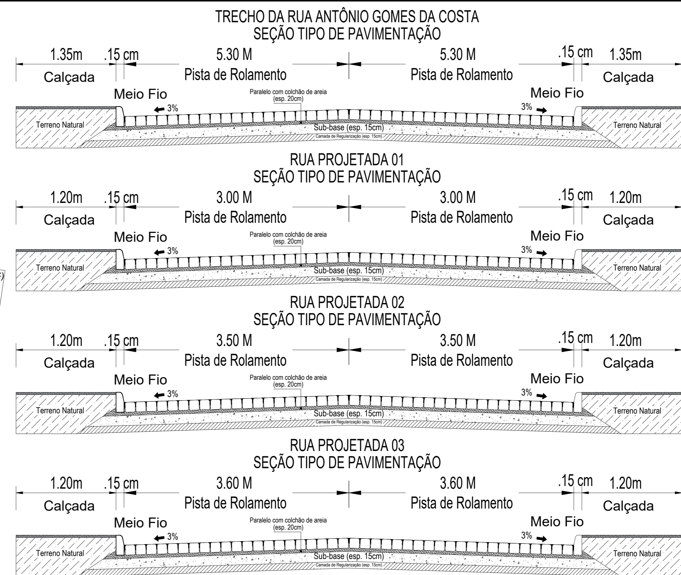
DETALHAMENTO DAS SEÇÕES ESCALA 1/75
