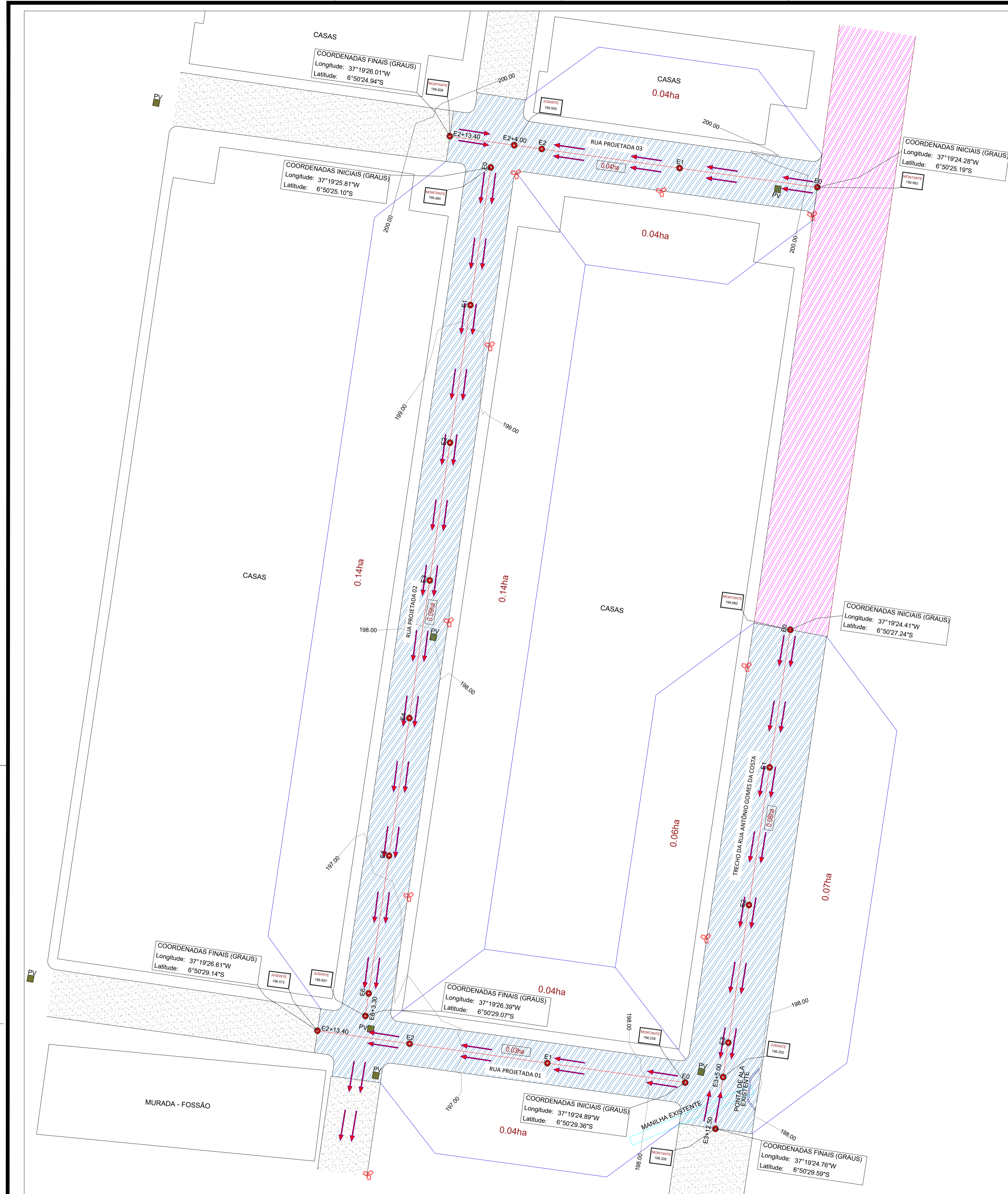
PLANTA DE SITUAÇÃO - RUAS GERAL ESCALA 1/250
