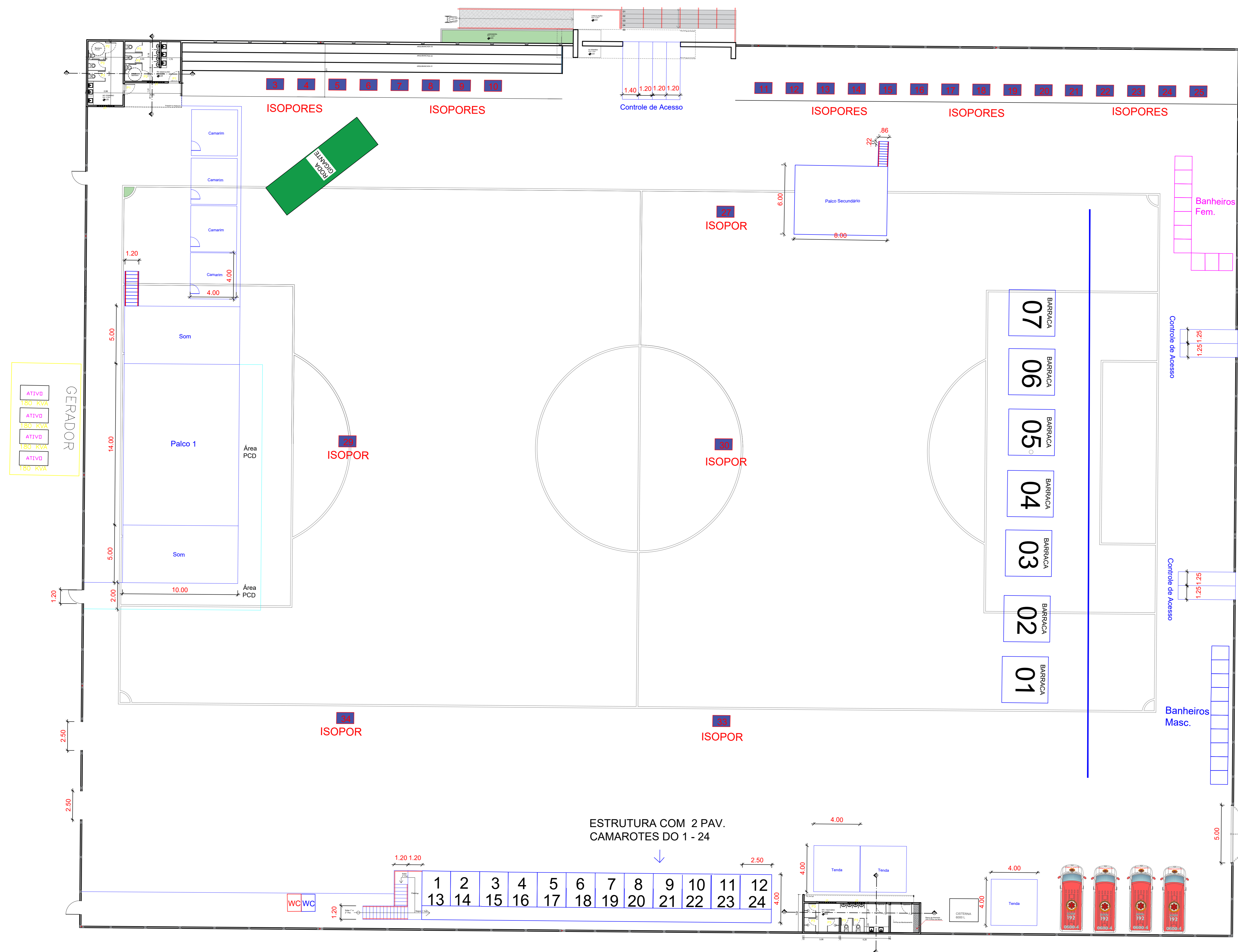
PLANTA BAIXA
