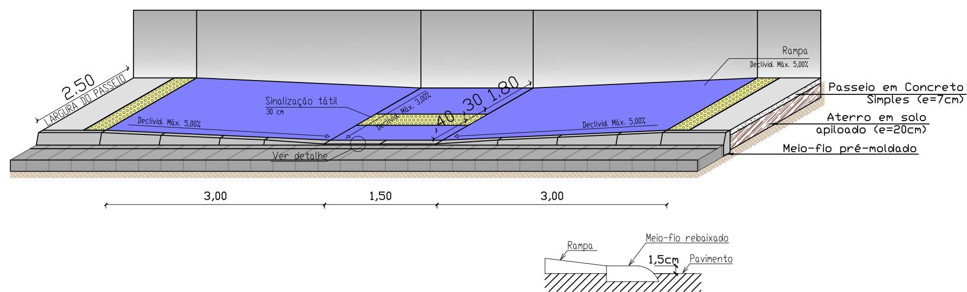
Detalhe – Rampa de acessibilidade 01 escala 1/50
