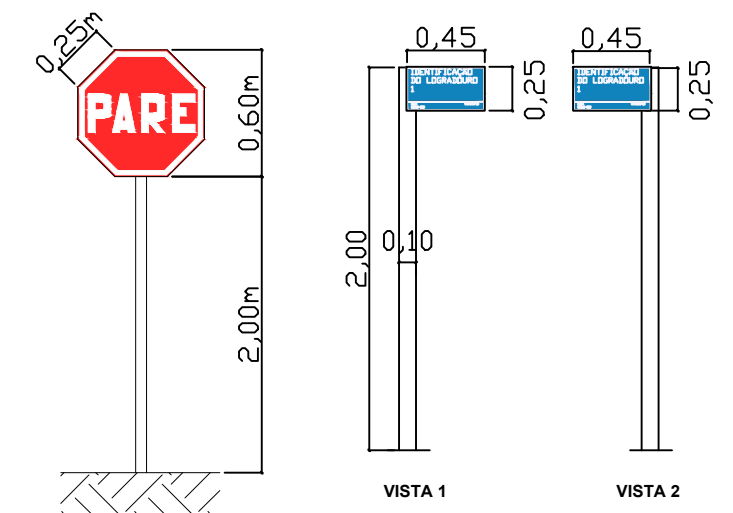
Detalhe de Placa de Sinalização escala → 1/400
