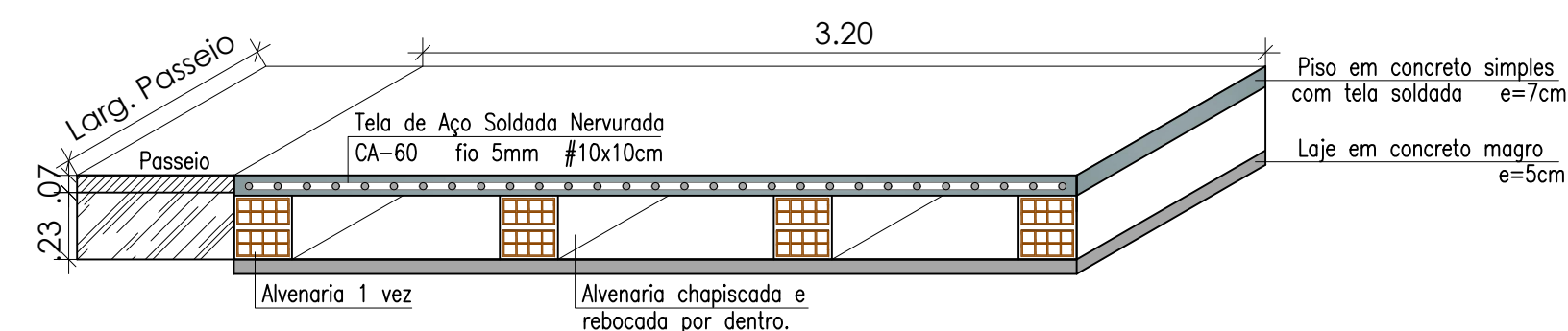
Detalhe 01 - Entrada Lateral de Água escala → 1/25
