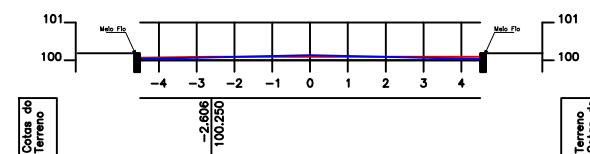
ESTACA 2
