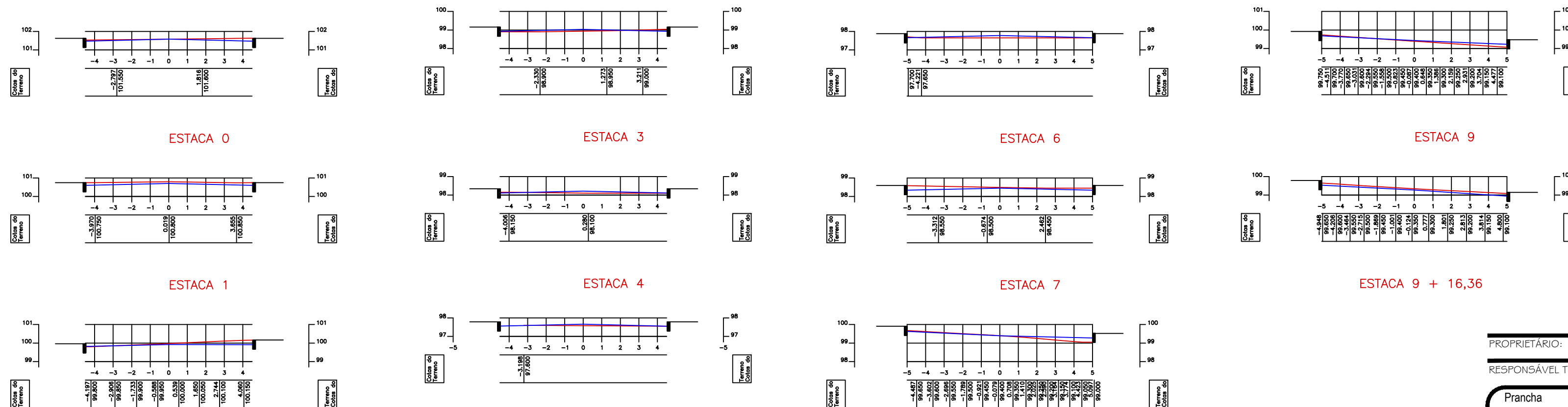
Seções Transversais escala 1:200
