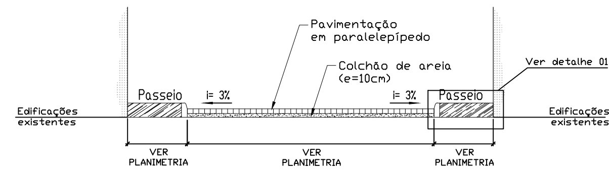
Seção Transversal tipo escala → 100
