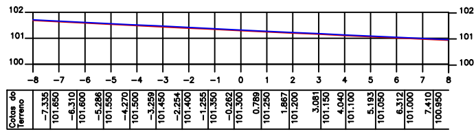
ESTACA 0
