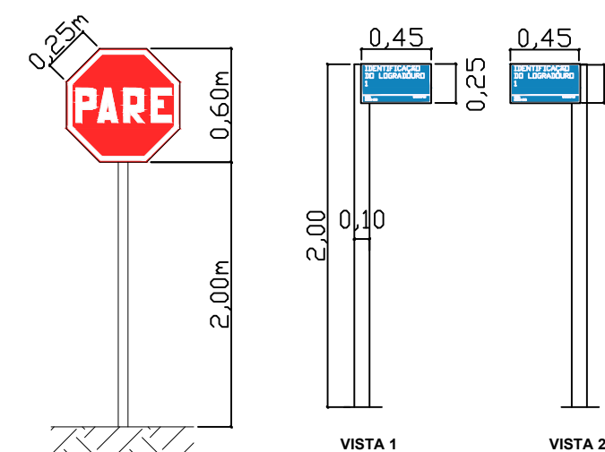
Detalhe de Placa de Sinalização escala 1/400
