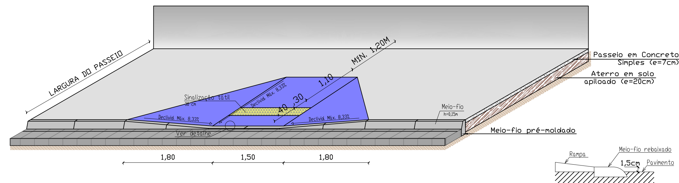
Detalhe – Rampa Acessível 02 escala 1/50
