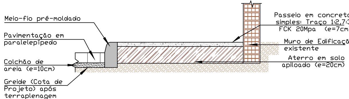
Detalhe 01 escala → 25
