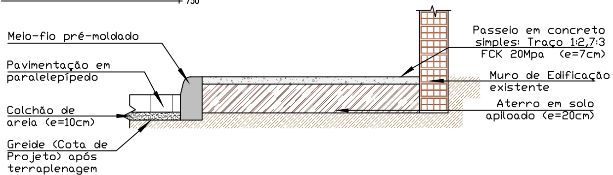
Detalhe 01 escala → 25
