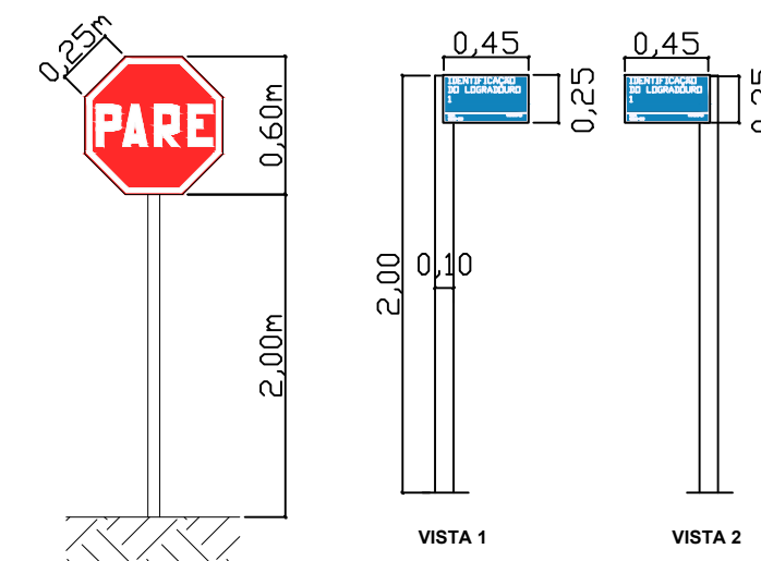
Detalhe de Placa de Sinalização escala → 1/400
