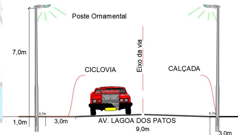
Figura 02: Detalhe construtivo na via
