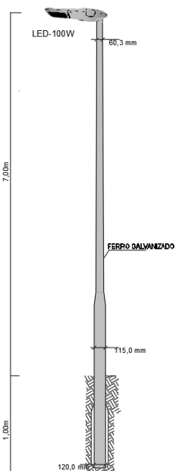
Figura 01: Detalhe dos postes ornamentais
