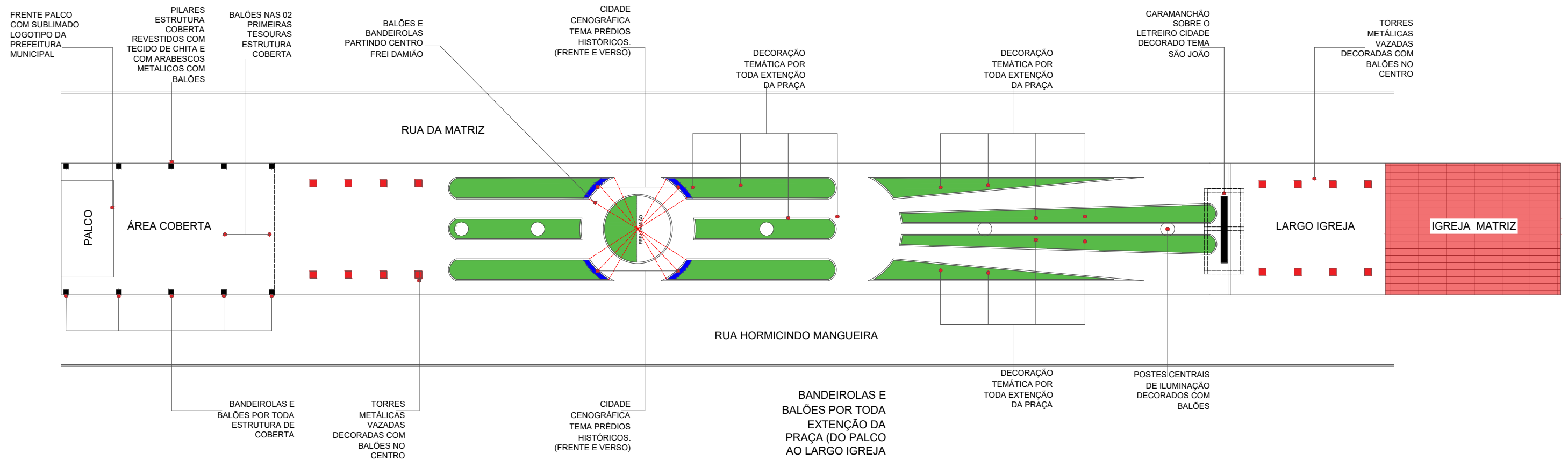
PLANTA LAYOUT SÃO JOÃO SANTANA DE MANGUEIRA - PB
