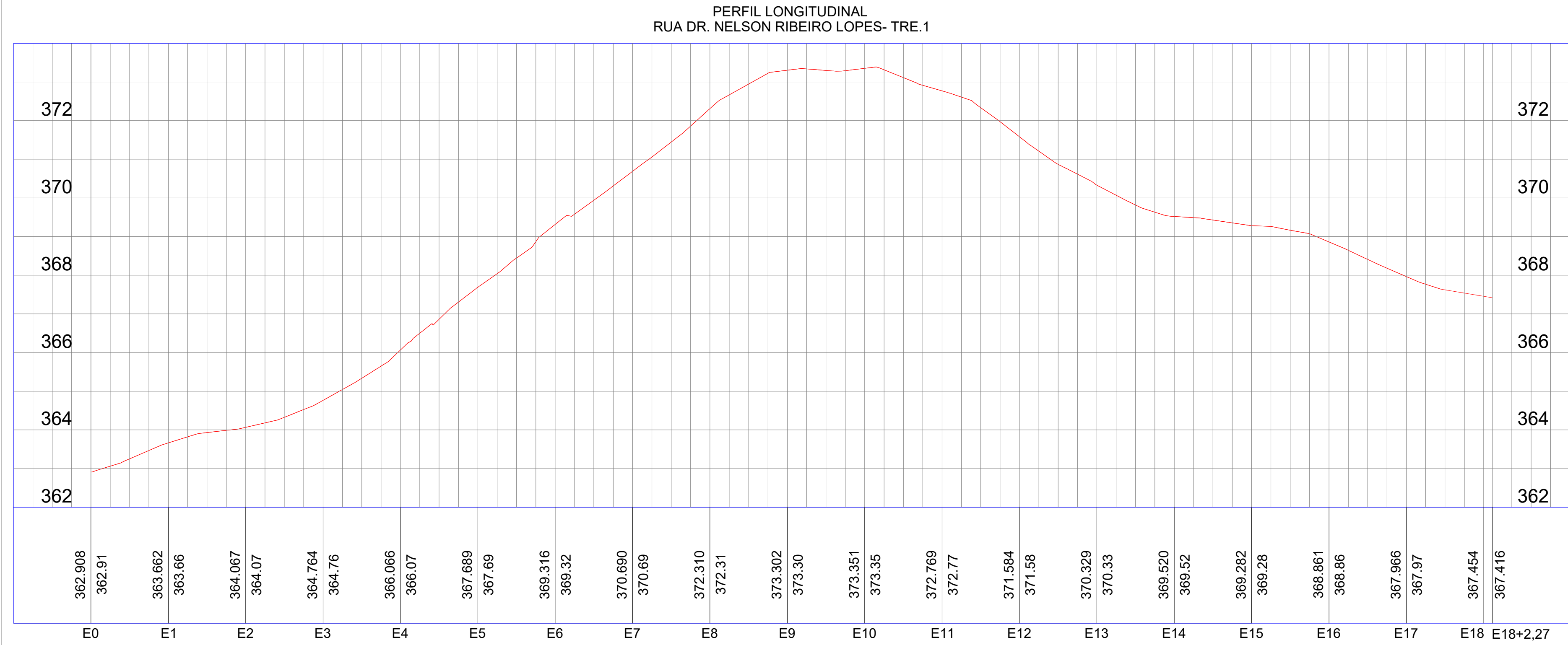
PERFIL LONGITUDINAL ESCALA 1/800
