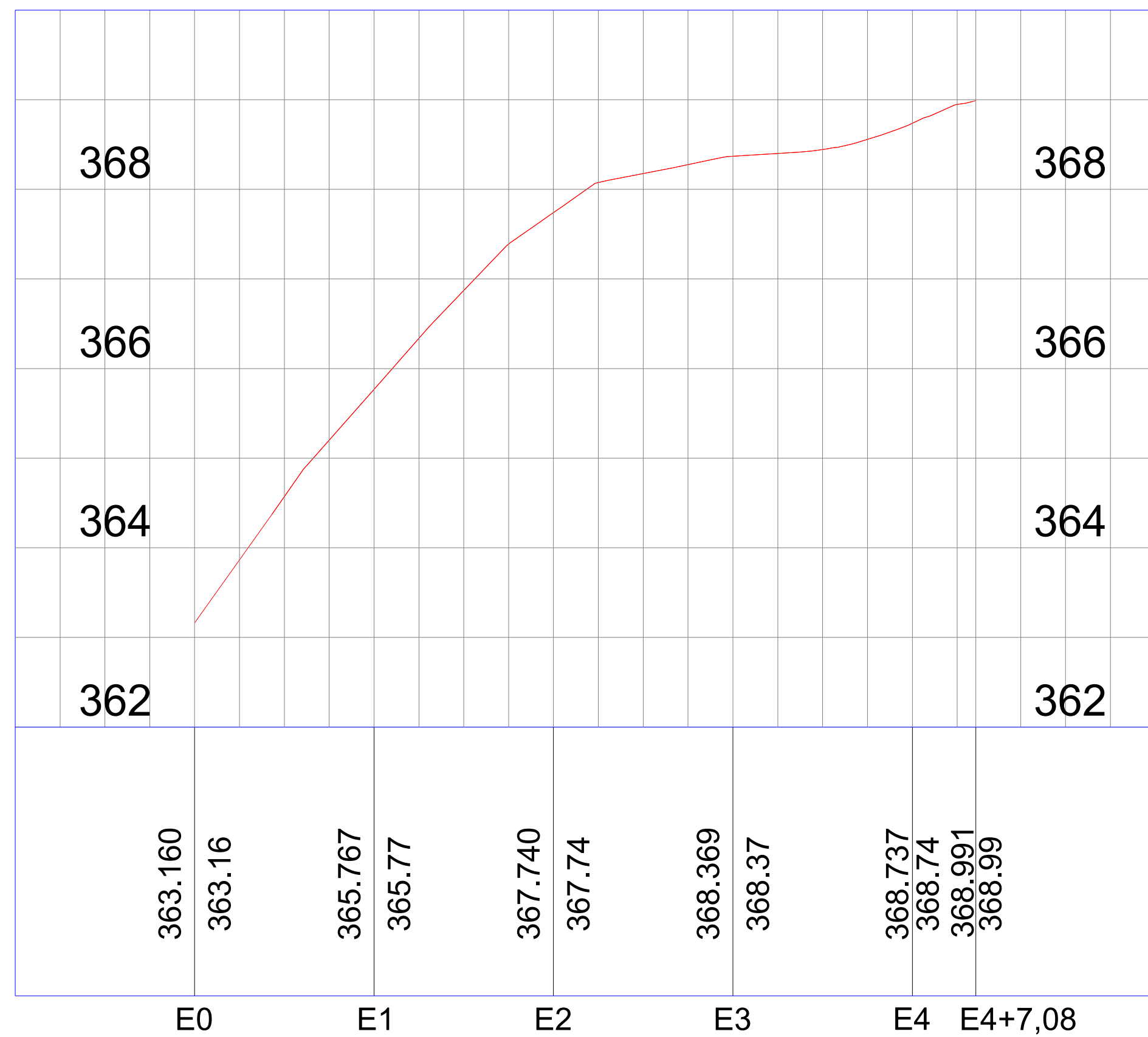
PERFIL LONGITUDINAL ESCALA _____ 1/800
