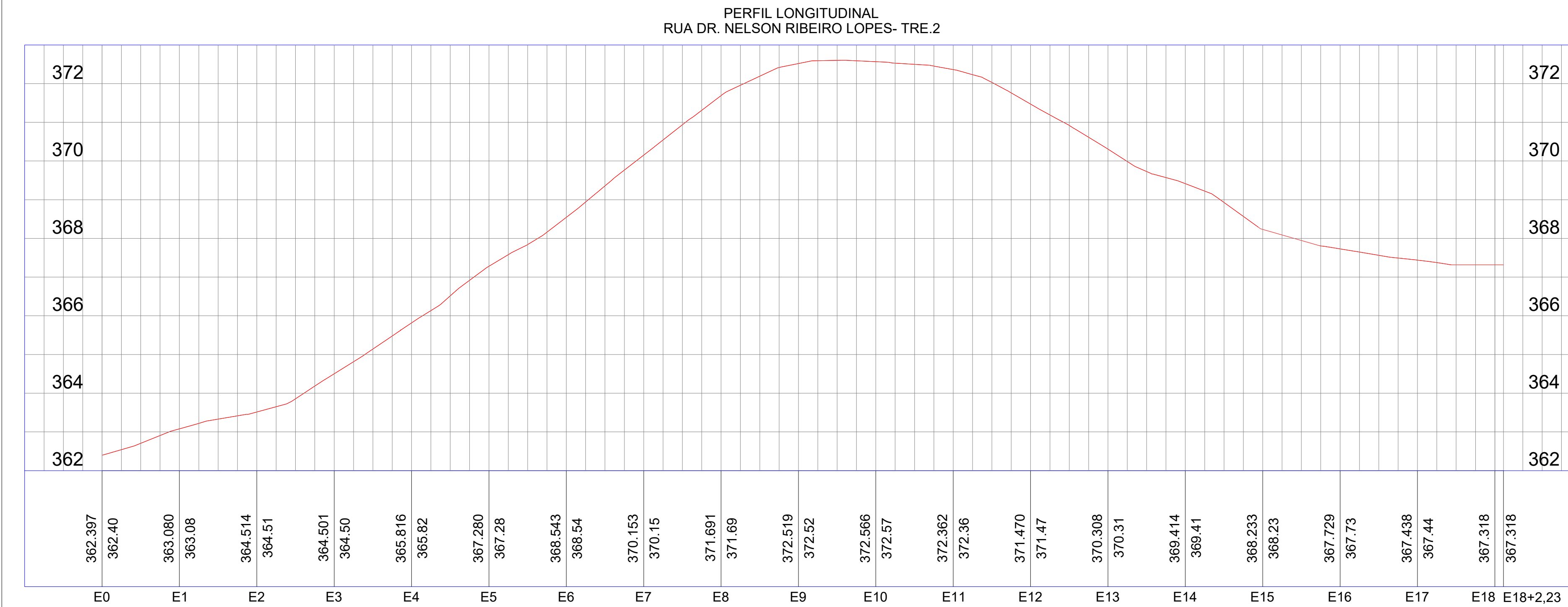
PERFIL LONGITUDINAL ESCALA 1/800
