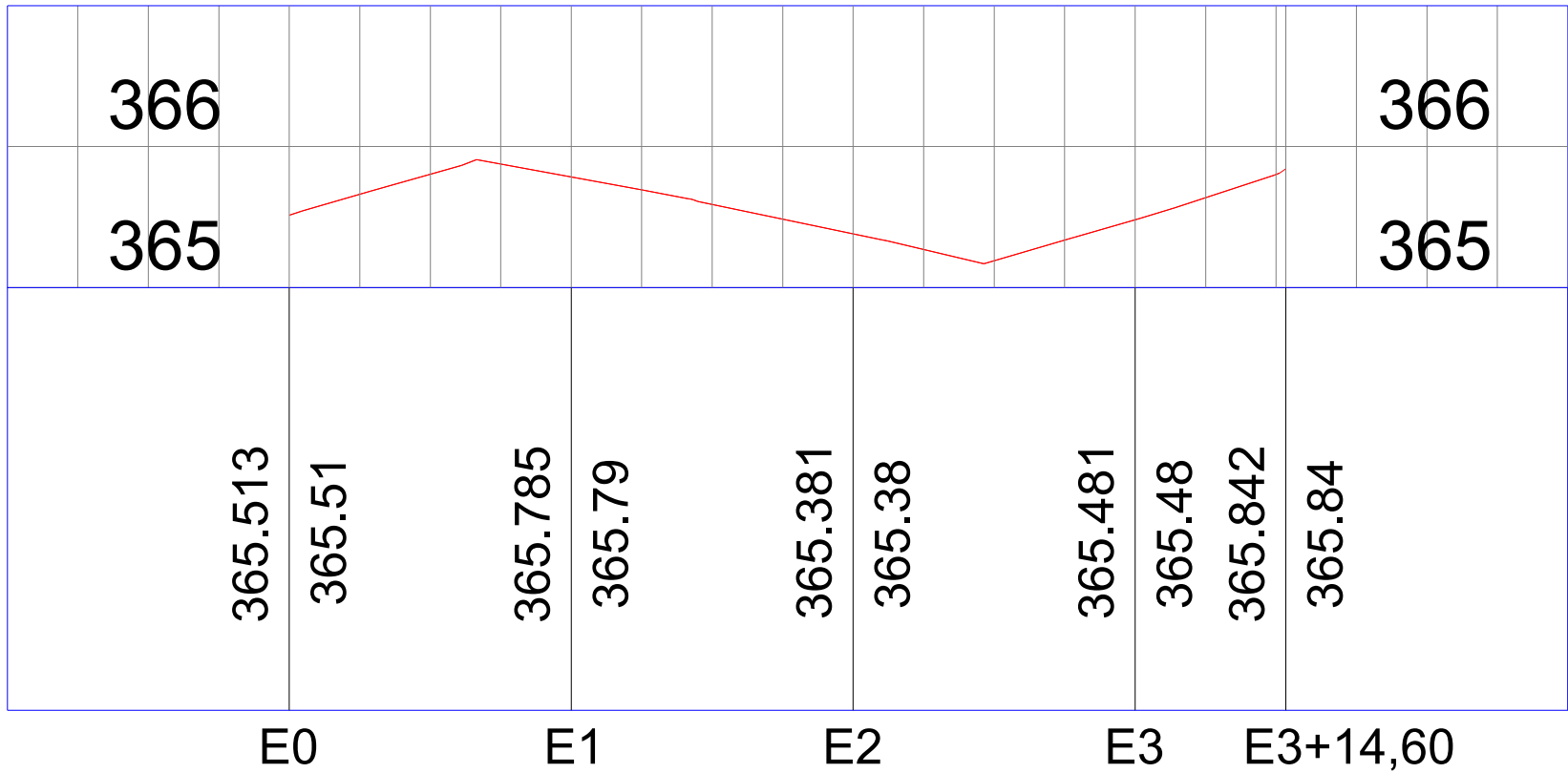
PERFIL LONGITUDINAL ESCALA 1/800
