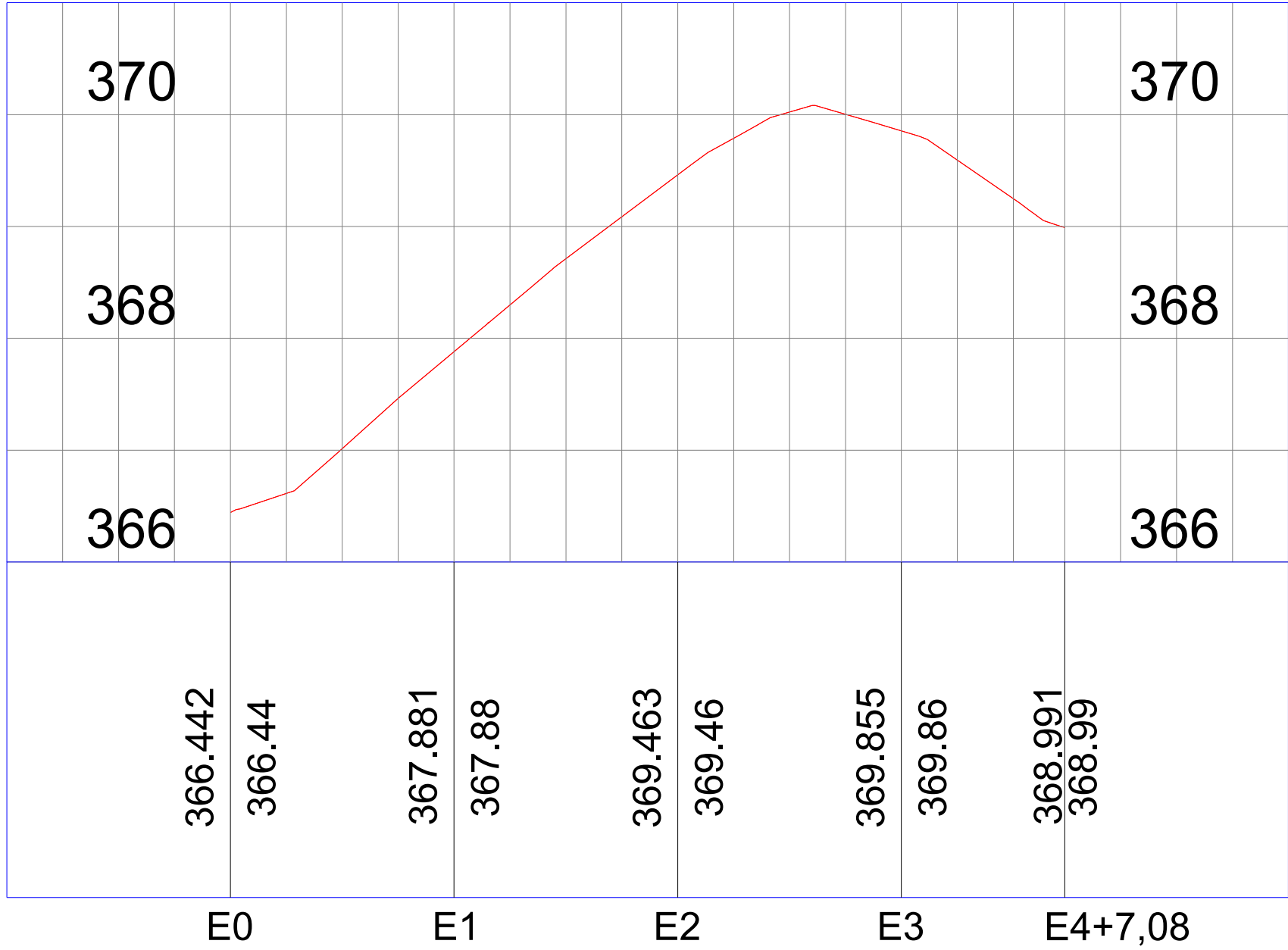
PERFIL LONGITUDINAL ESCALA 1/800
