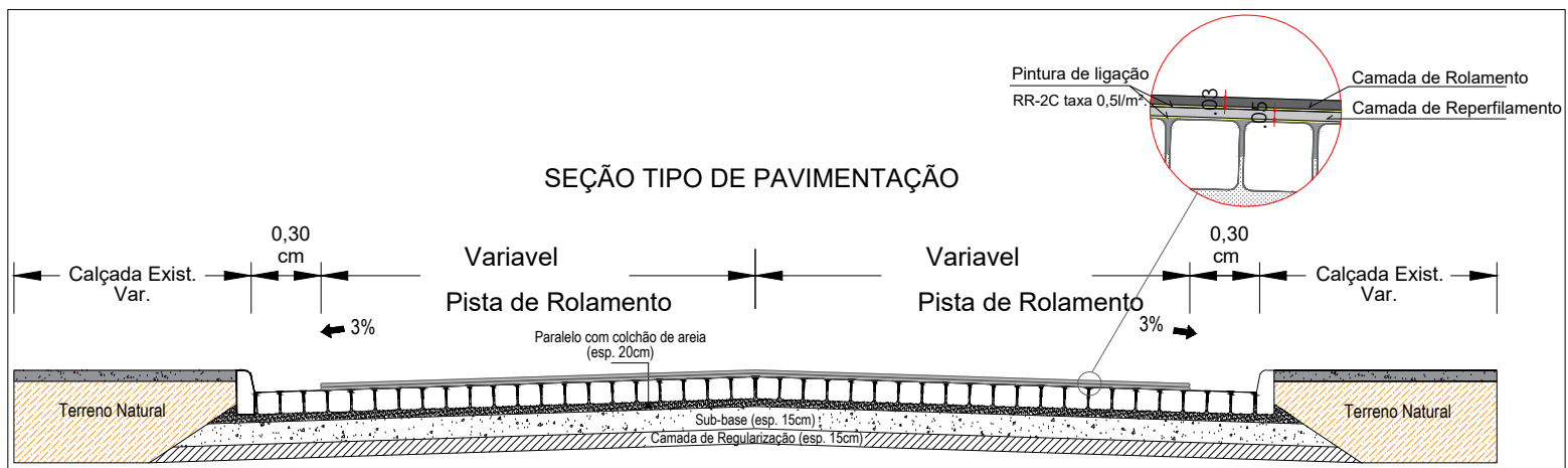
DETALHAMENTO DA SEÇÃO ESCALA 1/100
