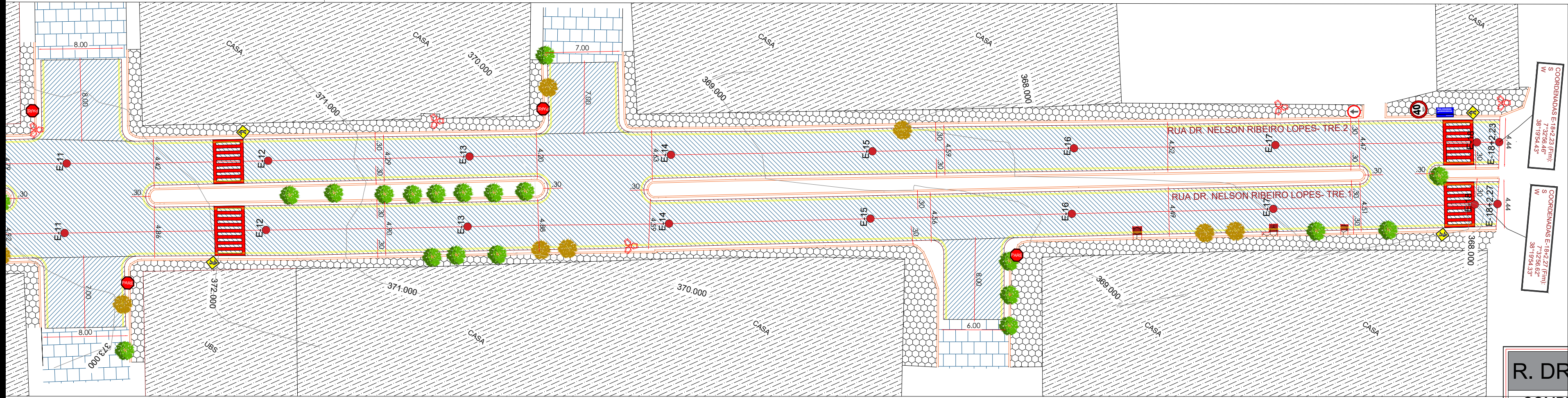
EST. E11 Á E18+2,27 PLANTA DE SITUAÇÃO ESCALA 1/300
