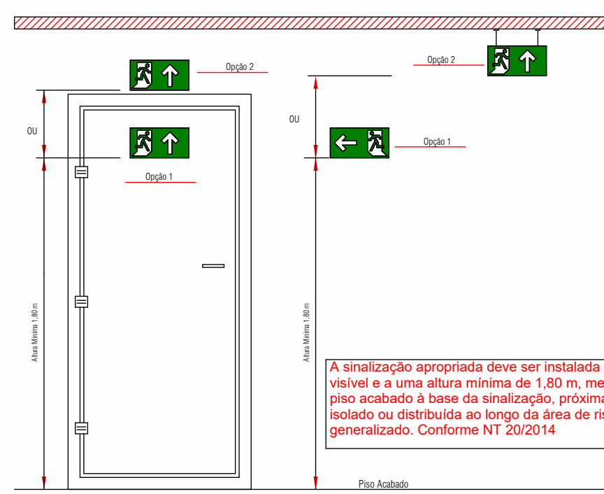
Instalação de Sinalização-PORTA/PAREDE/TETO 1 : 25
