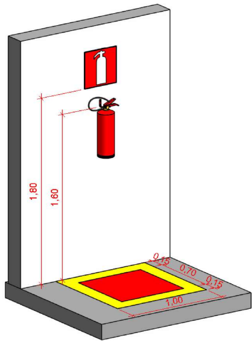
Extintor - Na parede com sinalização de Solo 1 : 20
