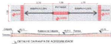
DETALHE DA RAMPA DE ACESSIBILIDADE
